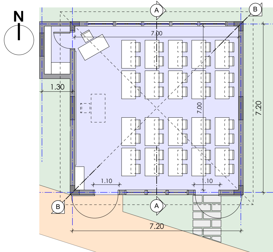
1 PLAN D'AMENAGEMENT 1:100
